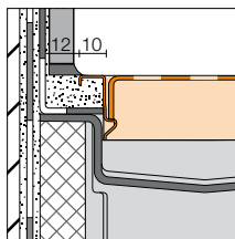
Obr. profilový rám
