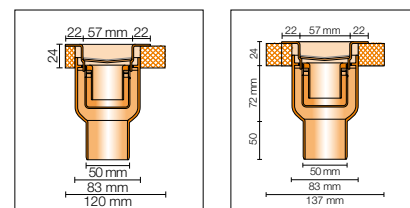
Průřez - montáž ke stěně
