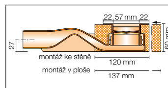
Průřez
