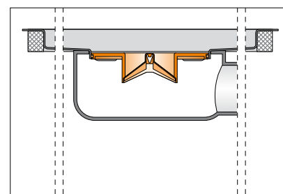
Podélný řez
