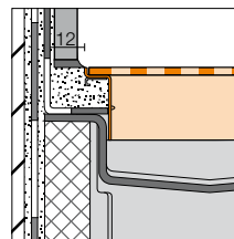
Obr. konturový rám
